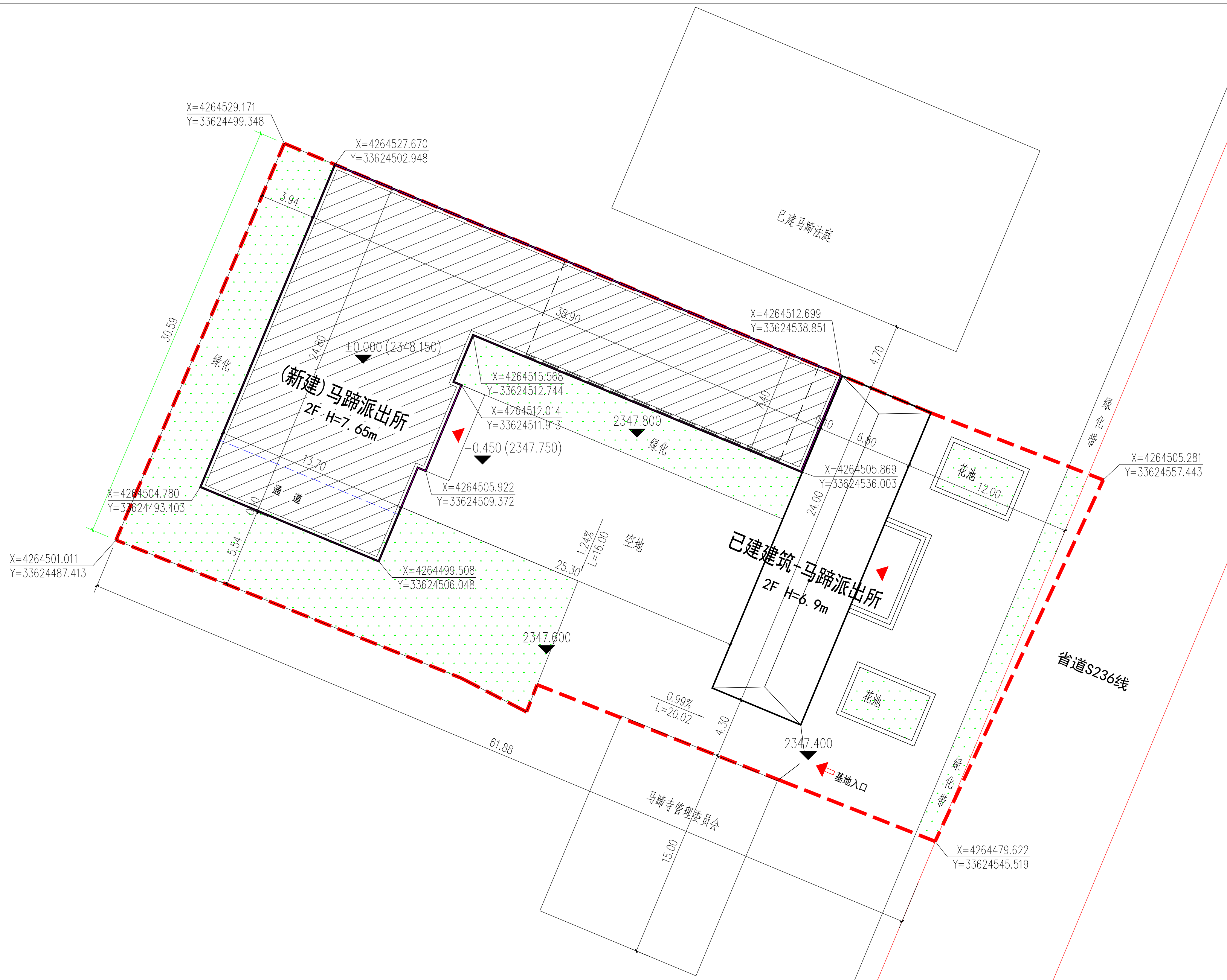
总平面布置图 1:200
