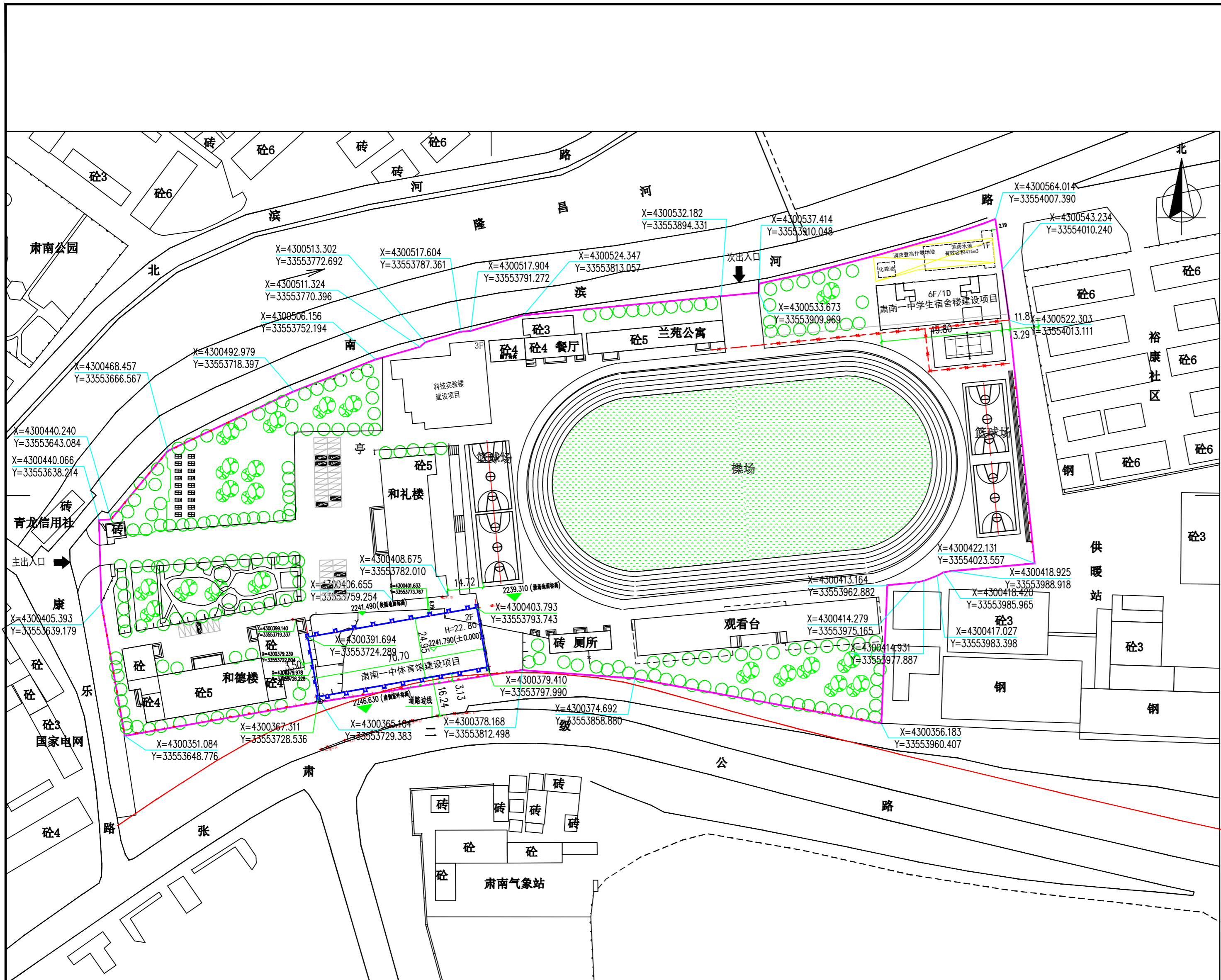
总平面布置图 1:1000
