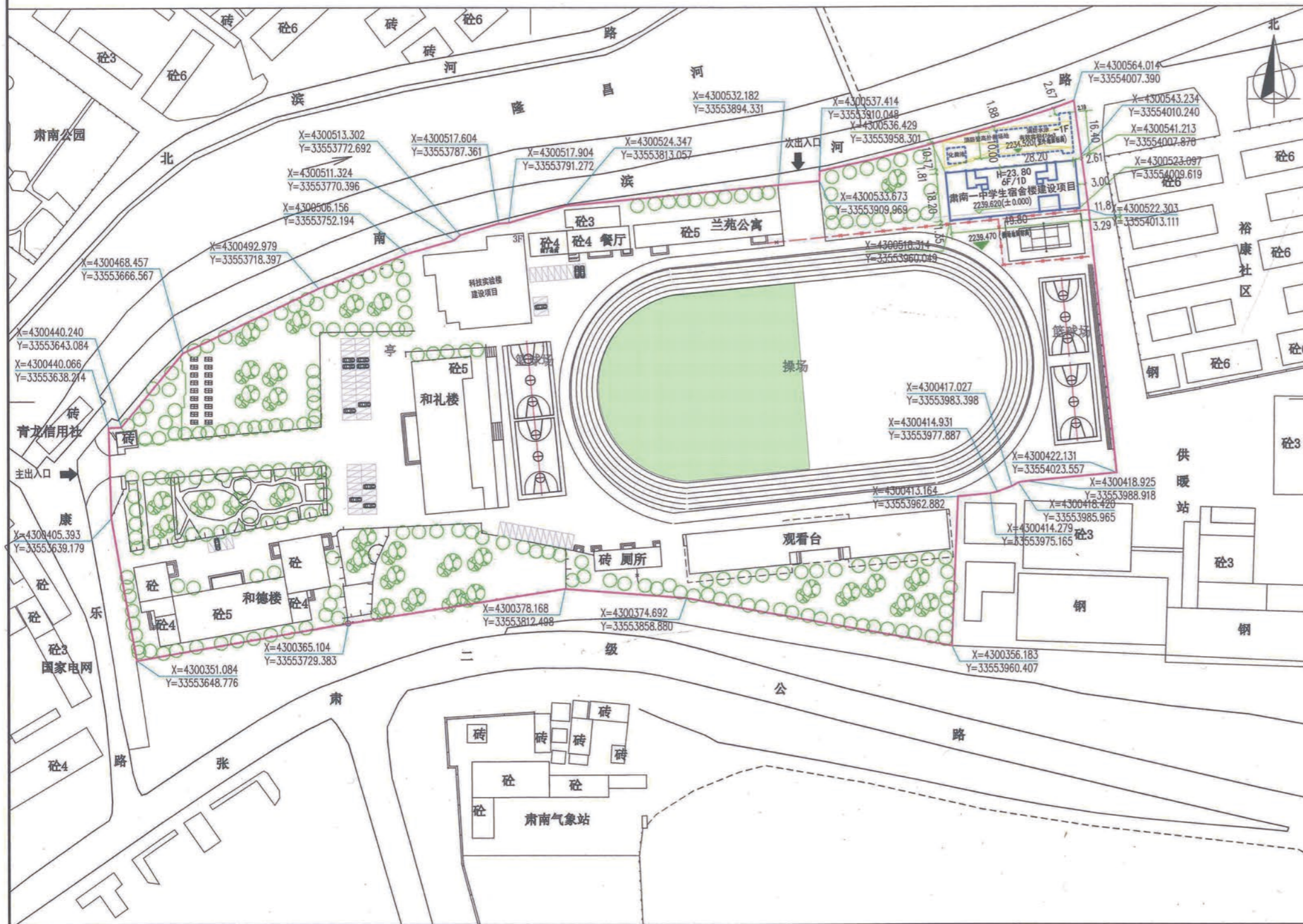
总平面布置图 1:1000
